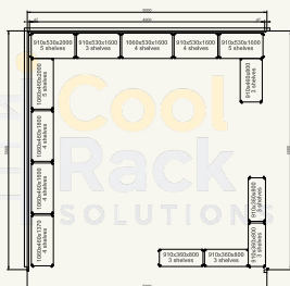
ΚΑΤΟΨΗ / PLAN
